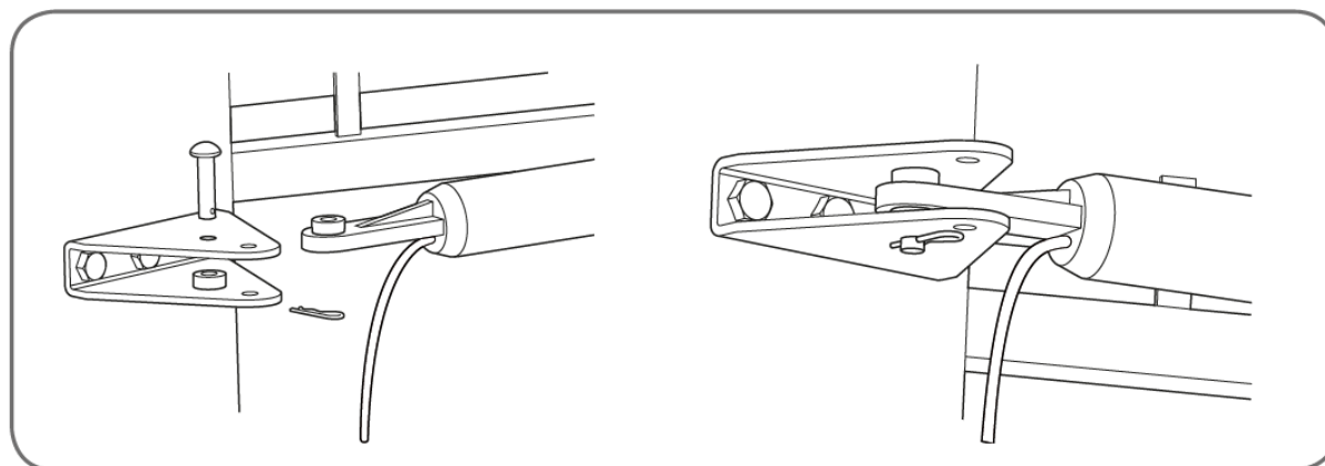
Assemblage du piston et de la patte pilier
