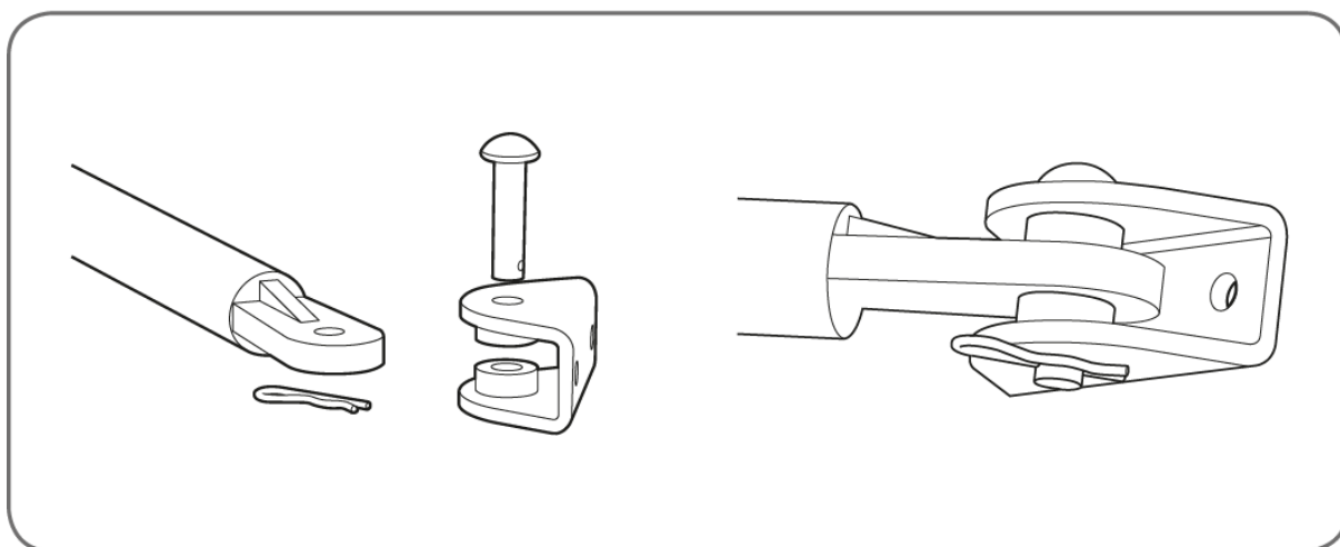
Assemblage du piston et de la patte pilier
